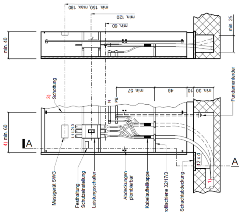
Schnitt A-A
