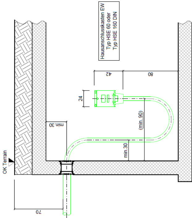
Schnitt A-A
